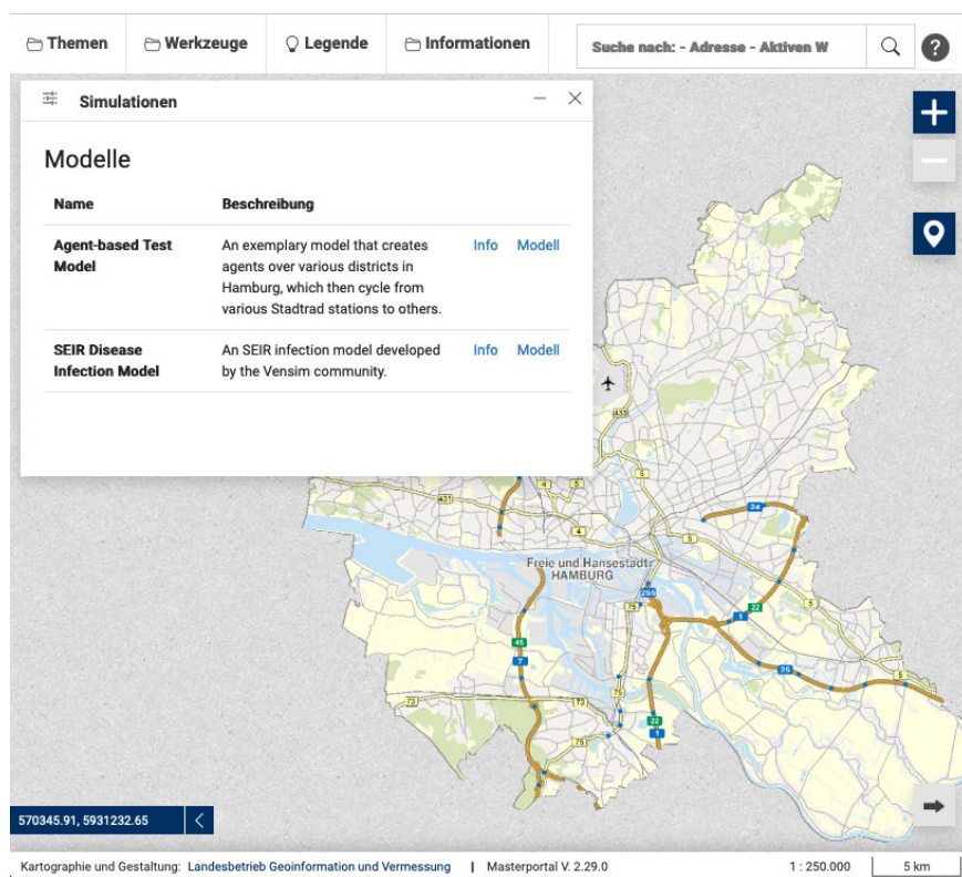
Abbildung 7: SimCo Übersichtsseite
